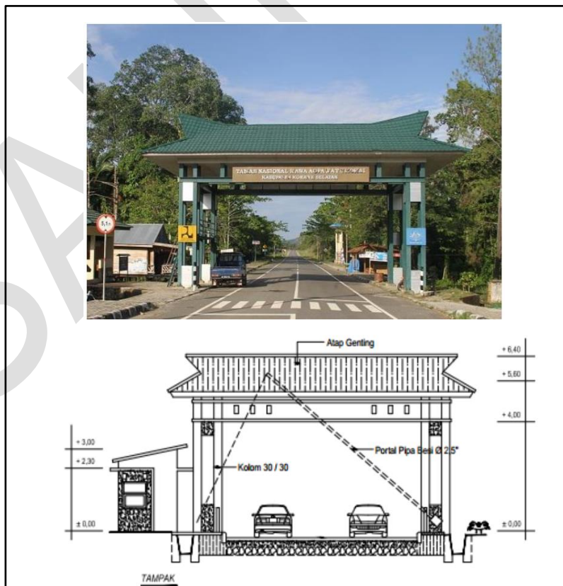
Gambar B.6 - Contoh desain pintu gerbang
