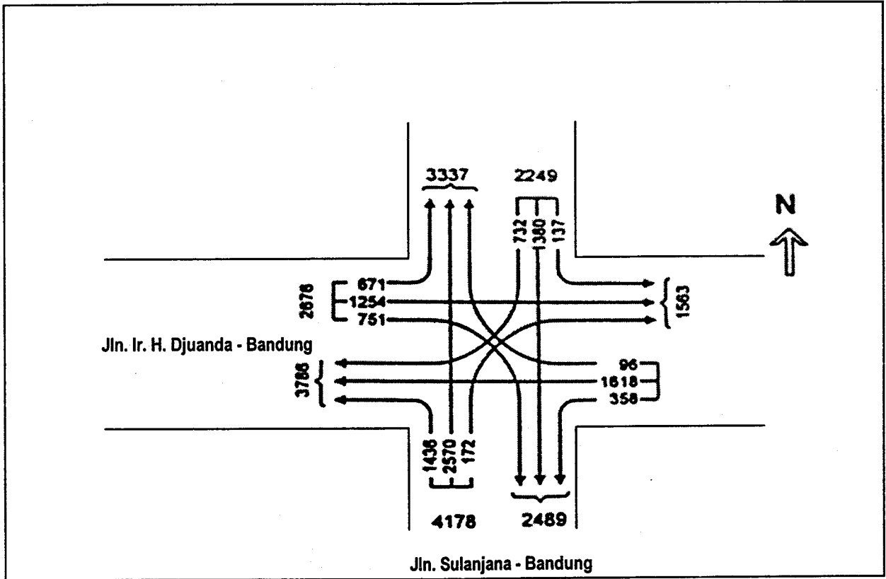
Gambar-G2 Contoh penyajian data lalu lintas pada persimpangan
