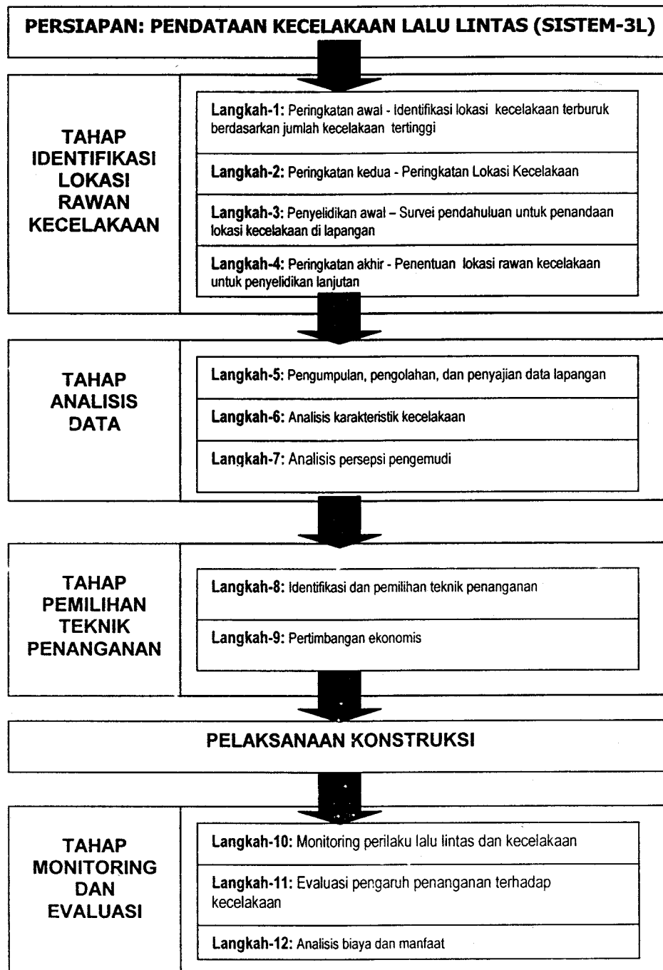
Gambar 3 Prosedur penyelidikan dan penanganan lokasi rawan kecelakaan
