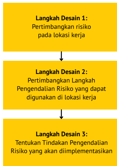
Gambar 1.6 Bagan alir penentuan Pengendalian Resiko
