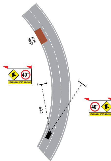
Gambar 3.2 Rambu-rambu peringatan dini diduplikasi bila area kerja terhalang tikungan
