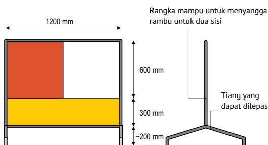
Gambar 3.1 Rangka rambu multi-pesan dibuat dari bahan metal hitam ringan
